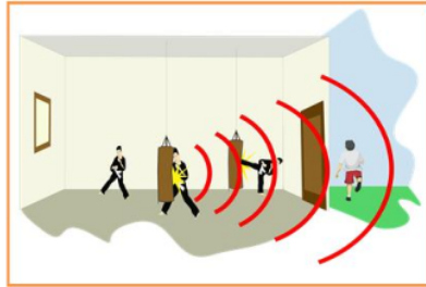
Gambar 3.5 Difraksi
